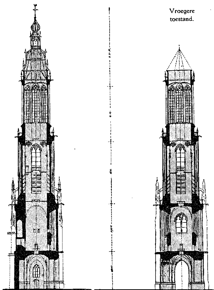
Afb.1. Tekeningen van de Cuneratoren van J.A.Snellebrand Getekend in 1915
