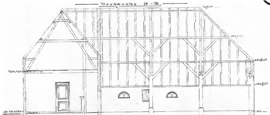
De Brijpot, lengte doorsnede 1915.
