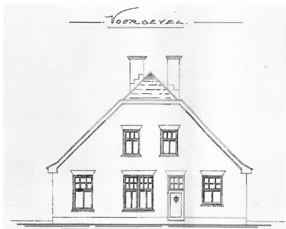
De Brijpot, bouwtekening, vooraanzicht 1918.
