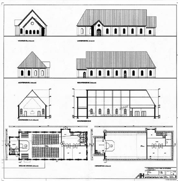
Bouwtekeningen voor de bouw van een nieuwe en grotere kerk.
