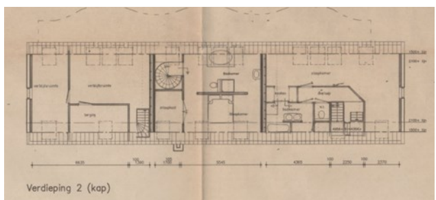
2 e verdieping van de appartementen
