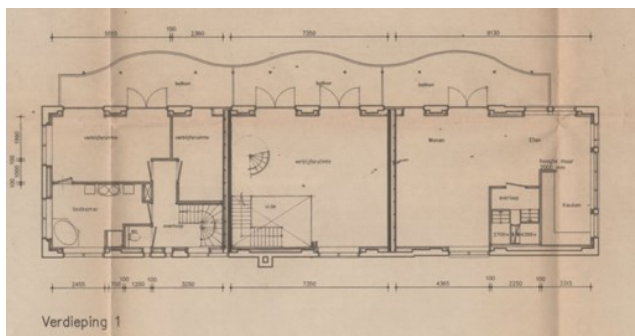
1 e verdieping van de appartementen met het balkon
